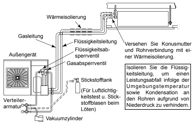
Beispiel für die Entleerung und Kältemittelauffüllung.
