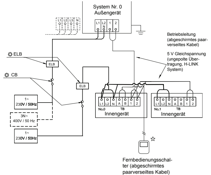
Unabhängige Stromversorgung des Außengeräts IVS und des Innengeräts (Beispiel)
