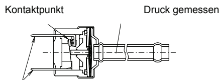
Aufbau des Hochdruckschalters
