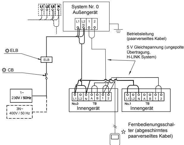
Stromversorgung vom Außengerät IVX zum Innengerät (Beispiel)
